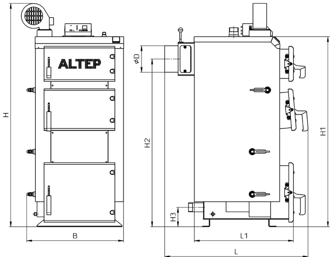
Рисунок 1 – Габаритне креслення котла типу КТ-1Е
